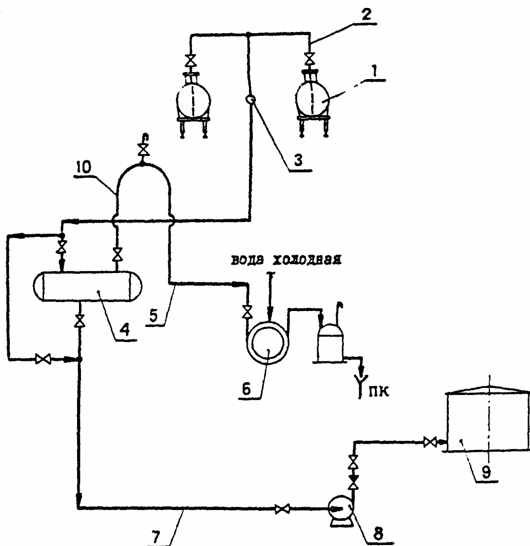
Принципиальная схема вакуумной системы слива 1 - цистерна; 2 - сливной стояк; 3 - всасывающий коллектор; 4 - вакуумсборник; 5 - вакуумная линия; 6 - вакуум-насос; 7 - всасывающий трубопровод; 8 - насос; 9 - резервуар; 10-гидравлический затвор
