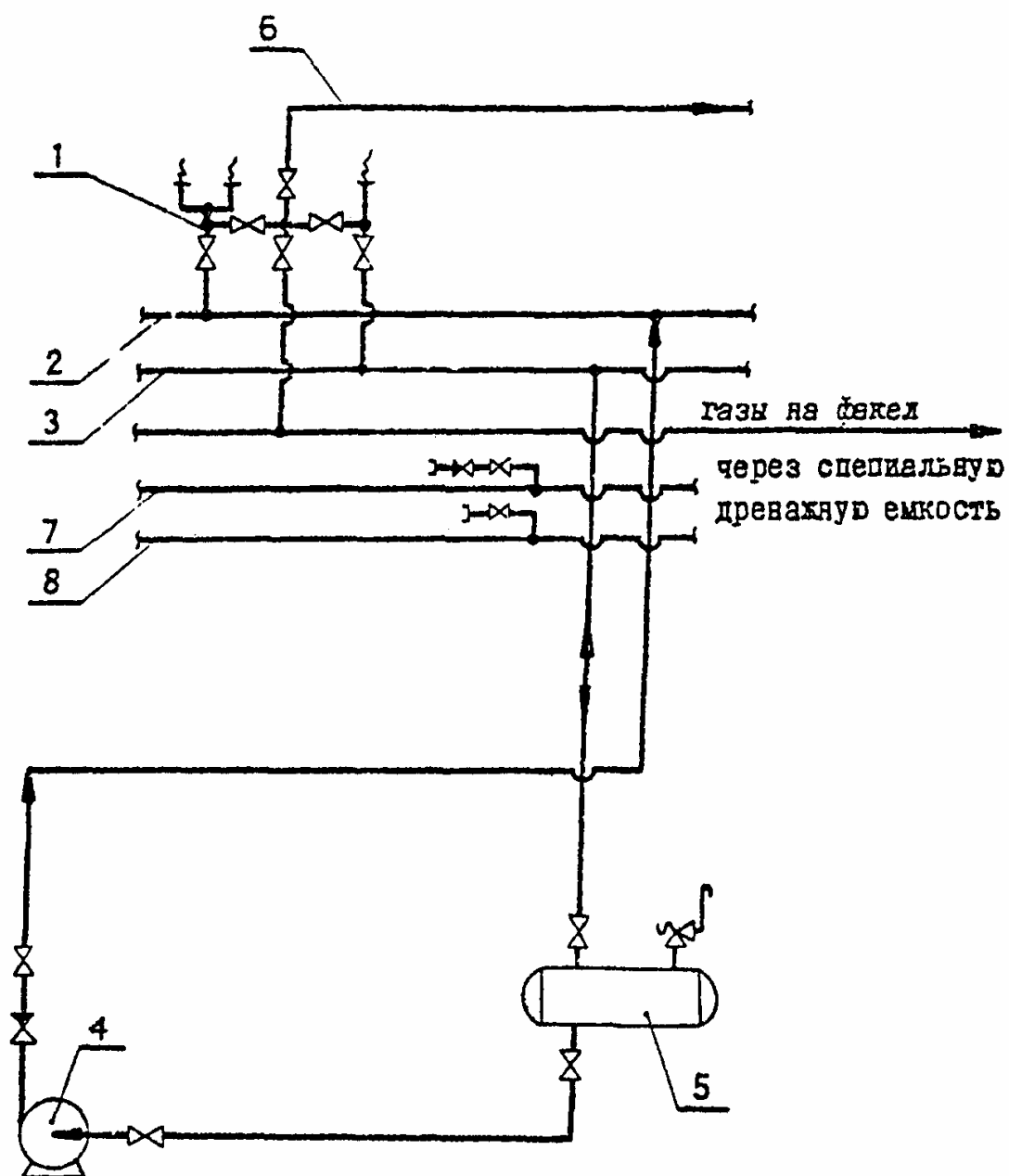
Схема налива сжиженных углеводородных газов без компрессорной установки
