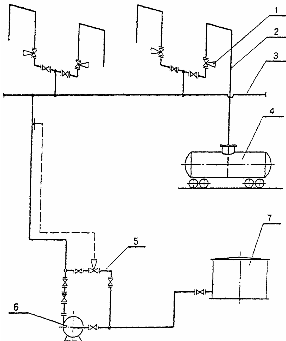
Схема налива светлых нефтепродуктов с пневматическим ограничителем уровня налива 1 - пневматический ограничитель, 2 - наливной стояк, 3 - напорный коллектор, 4 - цистерна, 5 - байпас, 6 - насос, 7 - резервуар
