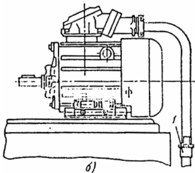
Рис. 74. Подвод трубы к электродвигателям 4 — 8-го габаритов. а — подвод сбоку электродвигателя; б — подвод со стороны вентилятора электродвигателя; 1 — разъемное соединение трубы.
