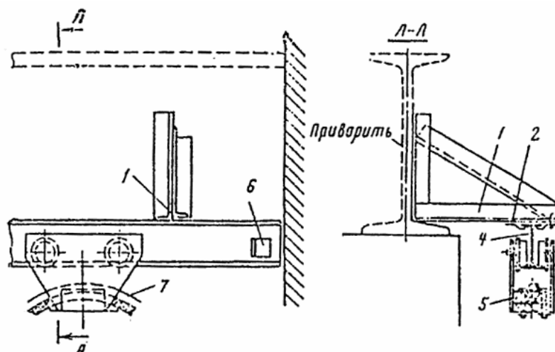
Рис. 106. Крепление двутавровой балки к подкрановому пути.
