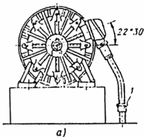
Рис. 74. Подвод трубы к электродвигателям 4 — 8-го габаритов. а — подвод сбоку электродвигателя; б — подвод со стороны вентилятора электродвигателя; 1 — разъемное соединение трубы.
