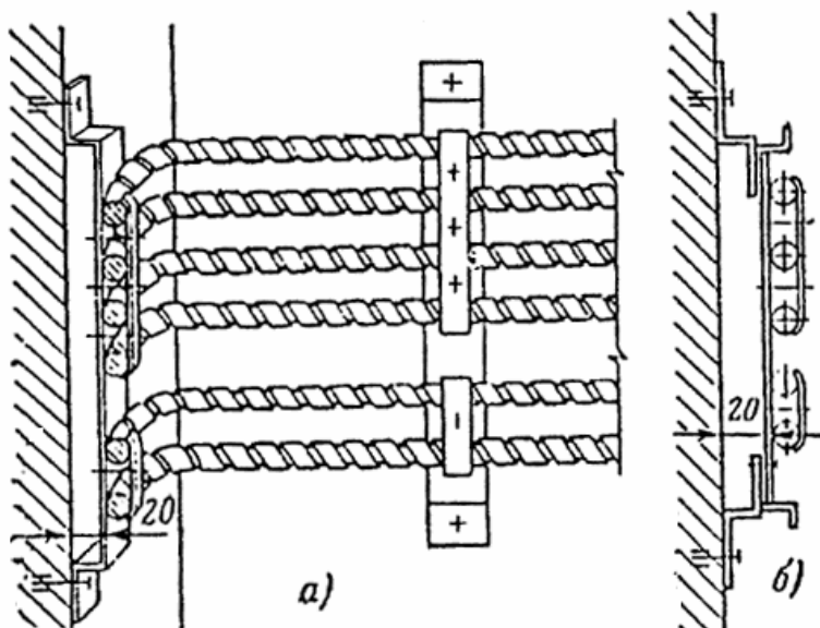
Рис. 10. Прокладка кабелей во взрывоопасных зонах классов В-II и В-IIa. а — по кабельным конструкциям с узкими горизонтальными поверхностями; б — по лоткам, установленным на ребро.
