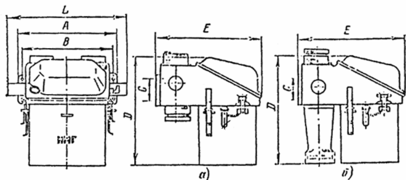
Рис. П9-1. Магнитные пускатели повышенной надежности против взрыва с маслonaполненными элементами.
