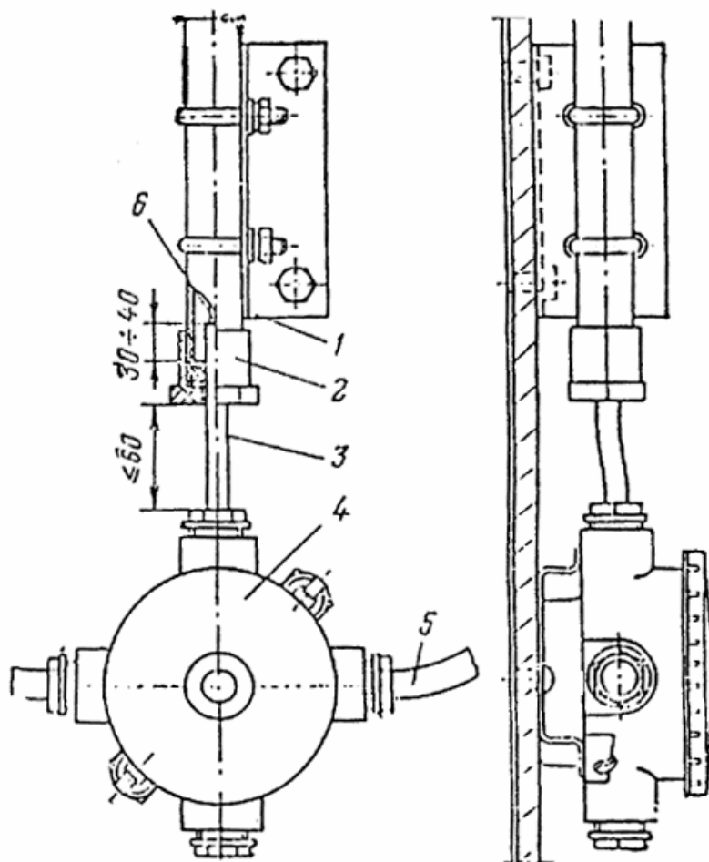
Рис. 101. Узел ввода провода ПРКС в коробку У409 от светильника с трубным кронштейном. 1 — трубный кронштейн; 2 — сальник трубный (для зон класса В-Па); 3 — трубка из поливинилхлоридного пластика; 4 — ответвительная коробка У409; 5 — кабель; 6 — провод ПРКС.
