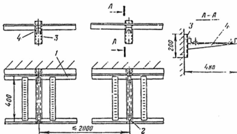
Рис. 9. Горизонтальная одноярусная установка лотков. 1 — лоток; 2 — прижим; 3 — стойка кабельная; 4 — полка кабельная.
