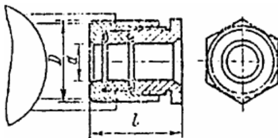
Рис. П7-2. Сальники ввертные по ТУ 36.108-72.
