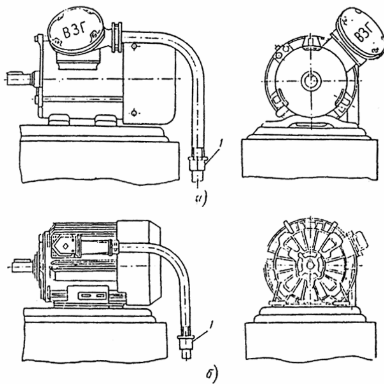
Рис. 73. Подвод труб к электродвигателям серии ВАО. a — подвод к электродвигателям 0 — 3-го габаритов; б — подвод к электродвигателям 9-го габарита; 1 — разъемное соединение трубы.
