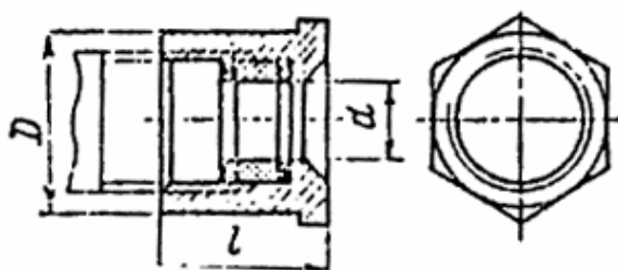
Рис. П7-1. Сальники трубные по ТУ 36.108-72.
