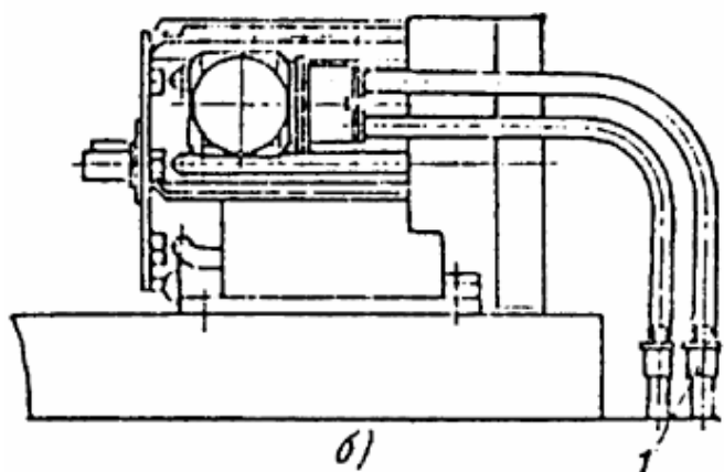
Рис. 75. Подвод труб к электродвигателям серии ВАО 315 — 450-го габаритов. а — подвод сбоку; б — подвод со стороны вентилятора; 1 — разъемное соединение трубы.
