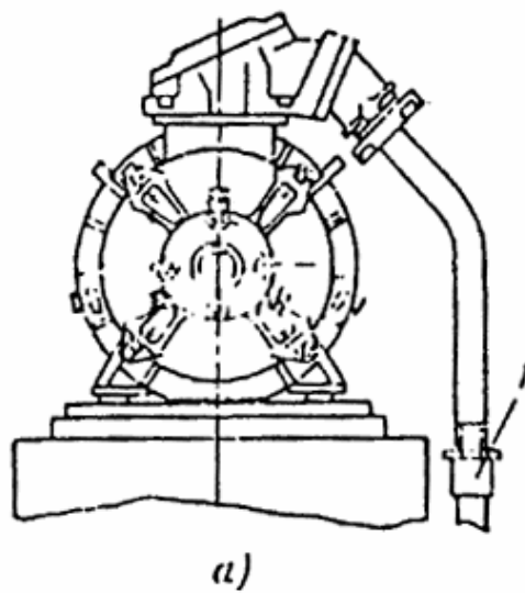
Рис. 73. Подвод труб к электродвигателям серии ВАО. a — подвод к электродвигателям 0 — 3-го габаритов; б — подвод к электродвигателям 9-го габарита; 1 — разъемное соединение трубы.
