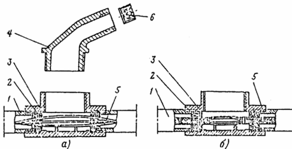
Рис. 37. Подготовка коробки КПР для выполнения разделительного уплотнения. а — крышка с пробкой и корпус с проложенными одножильными проводами и выполненной набивкой из джута; б — корпус с проложенным многожильным проводом ПРТО со снятой хлопчатобумажной оплеткой и выполненной набивкой из джута; 1 — трубопровод; 2 — набивка из джута или асбестового шнура; 3 — корпус; 4 — крышка; 5 — провод; 6 — пробка.
