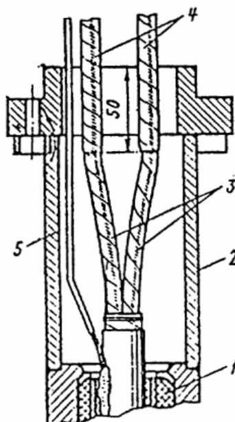
Рис. 53. Подготовка кабеля для заливки кабельной массой в кабельной муфте вводного устройства.
