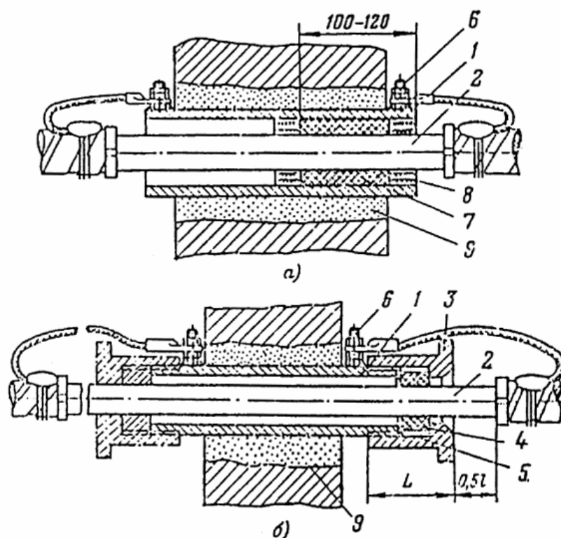
Рис. 11. Проходы кабелей сквозь внутренние стены помещений.
