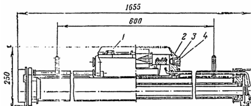
Рис. 92. Светильник повышенной надежности против взрыва НОГЛ-80.
