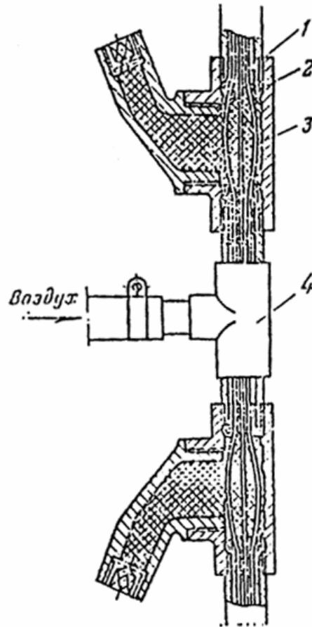
Рис. 35. Устройство разделительных уплотнений с локальным испытанием в коробках КПР. 1 — коробка; 2 — джгут или асбестовый шнур; 3 — уплотнительный состав УС65; 4 — тройник по ГОСТ 8949-59.
