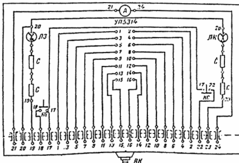
Рис П9-6. Электрическая схема колонки управления К-3Г.
