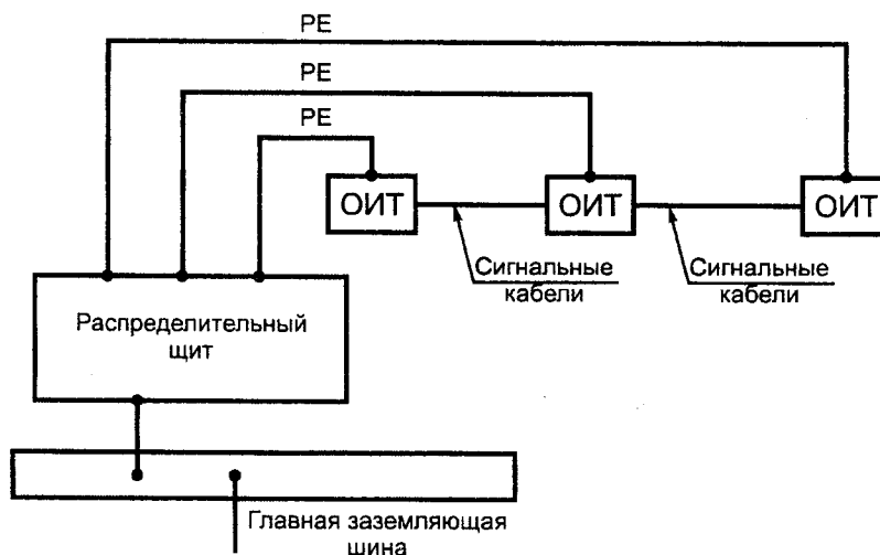
Рисунок В.1 — Радиально подсоединенные защитные проводники
