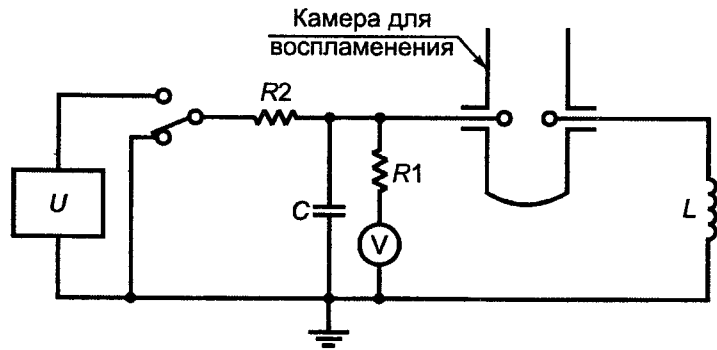
U — источник напряжения постоянного тока; C — конденсатор; R1 — резистор (развязывающее сопротивление); R2 — токоограничивающий резистор; V — электростатический вольтметр; L — индуктивность 1 мГн
