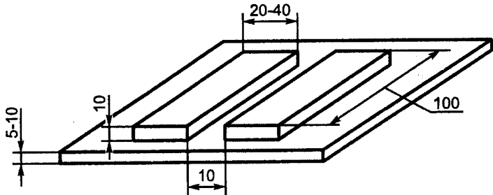
Рисунок 1 — Стенд для испытаний
