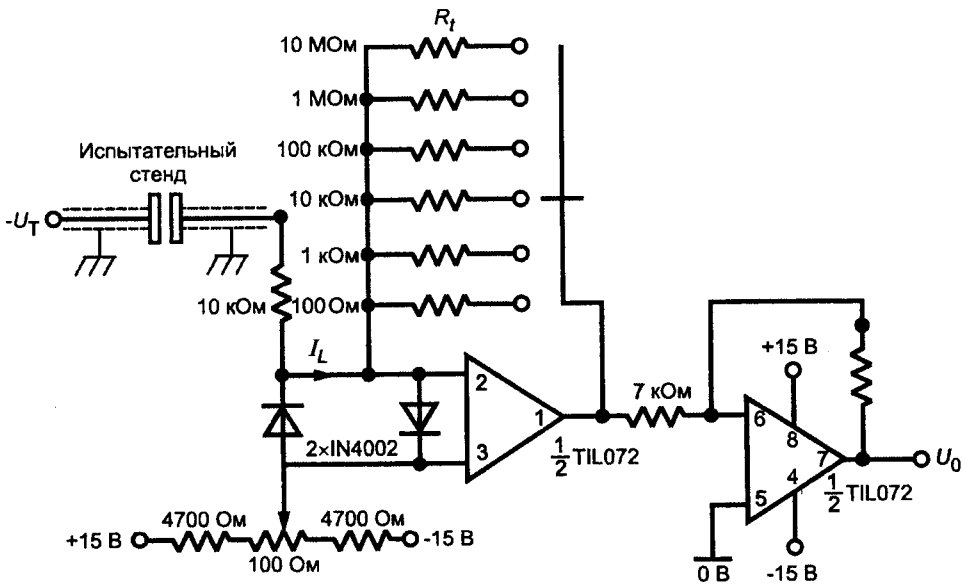
Рисунок 1 — Стенд для испытаний
