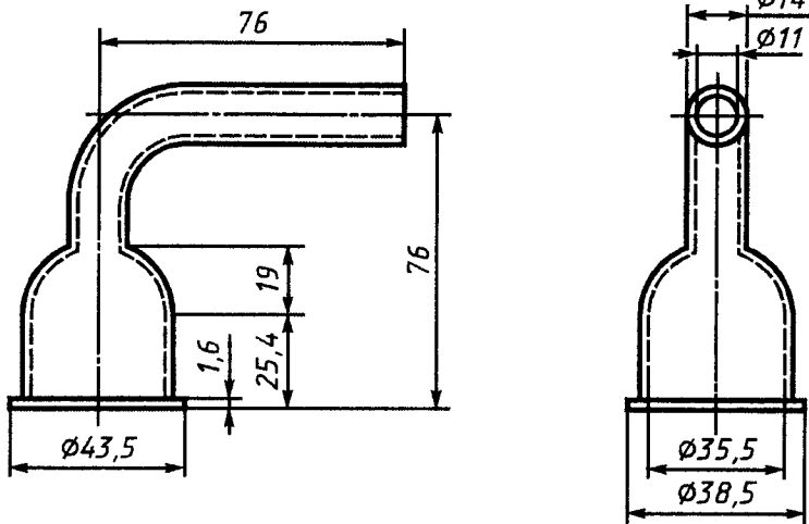
Дет. 4
