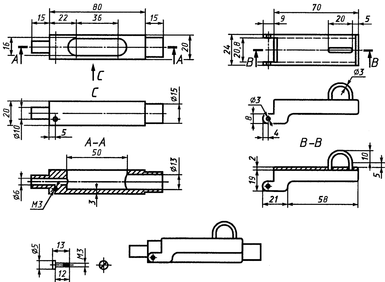
Дет. 30
