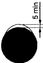
Рисунок А.1b — Чрезмерный слой пыли, имеющий температуру самовоспламенения менее 250 °С, на верхней поверхности оборудования
