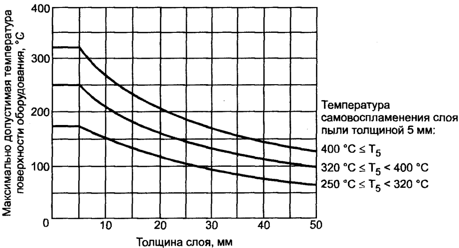
Рисунок 1 — Максимально допустимая температура поверхности в зависимости от толщины слоя пыли
