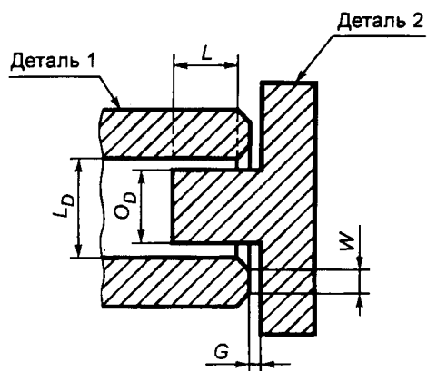
Рисунок 3 — Цилиндрическое соединение
