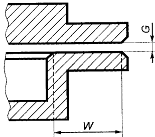
Рисунок 2 — Плоское соединение
