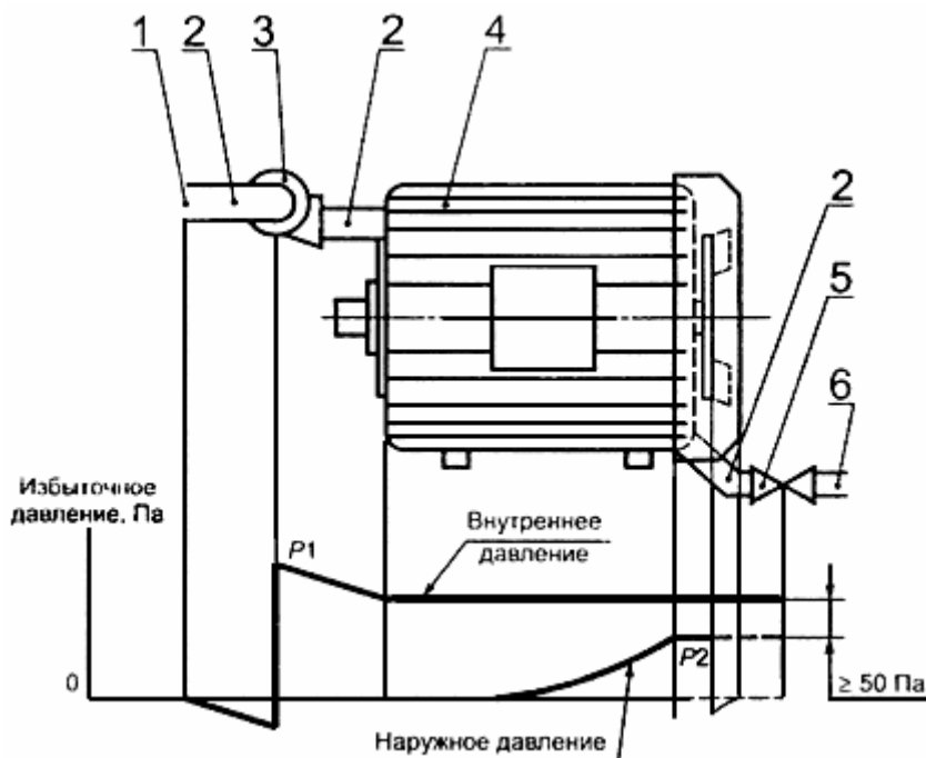
Рисунок В.3 - Оболочки под давлением с компенсацией утечки - вращающаяся электрическая машина с внутренним вентилятором
