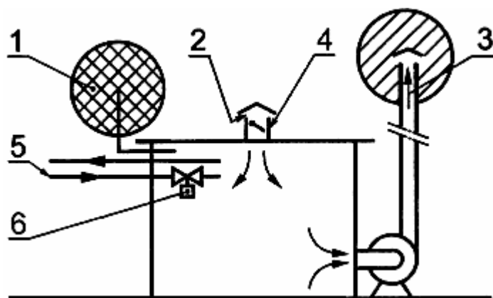
1 - вытяжная труба отбора проб; 2 - вход воздуха для вентиляции; 3 - выход воздуха из помещения; 4 - запорное устройство; 5 - контуры отбора проб; 6 - запорный кран Рисунок А.3 - Помещение для анализаторов во взрывобезопасной зоне (вытяжная система вентиляции)
