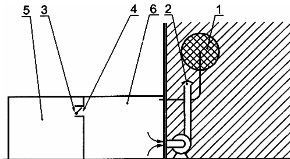
1 - вытяжная труба отбора проб; 2 - выход воздуха из помещения; 3 - запорное устройство; 4 - вход воздуха; 5 - служебное помещение; 6 - помещение для анализаторов Рисунок А.2 - Помещение для анализаторов в существующем сооружении
