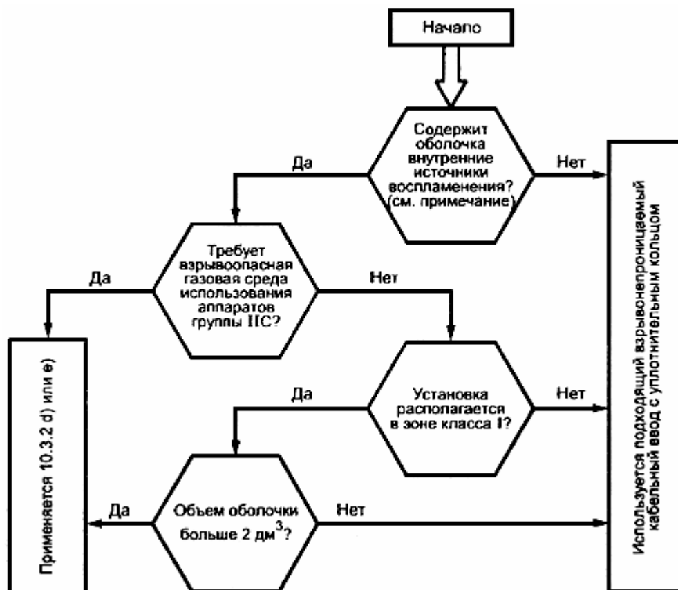
Рисунок 1 - Схема выбора кабельного ввода во взрывонепроницаемые оболочки для кабелей в соответствии с 10.3.2 b)
