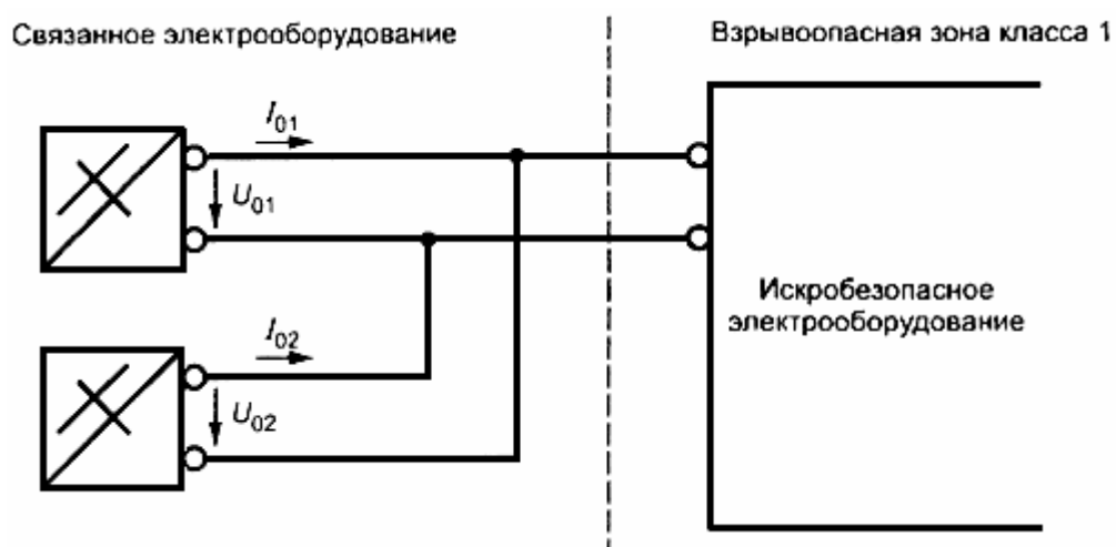
Рисунок В.2 - Параллельное соединение.
