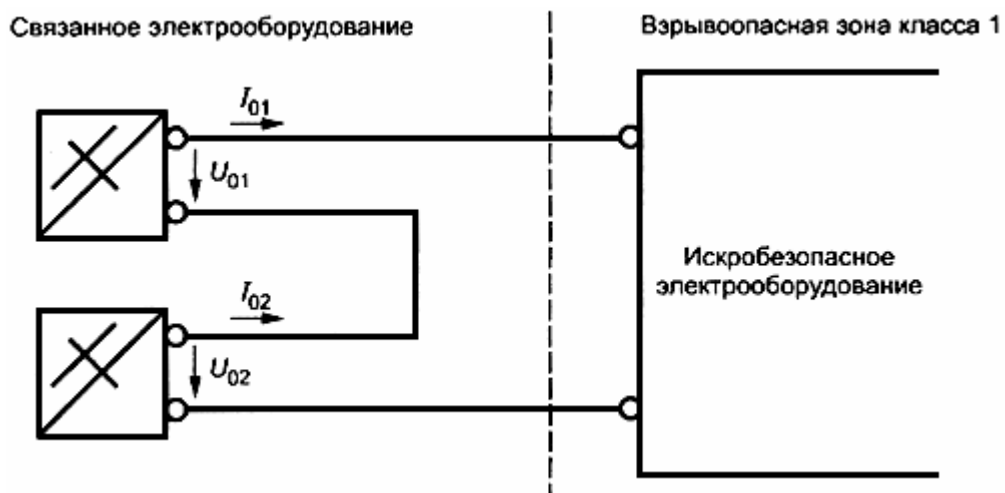
Рисунок В.1 - Последовательное соединение.
