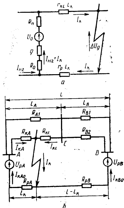
а — одностороннее питание контактной сети; б — двустороннее питание контактной сети на двухпутном участке с постом секционирования
